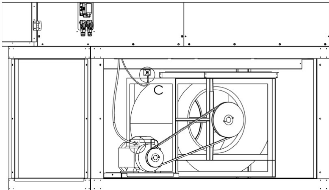
С - Датчик температуры
