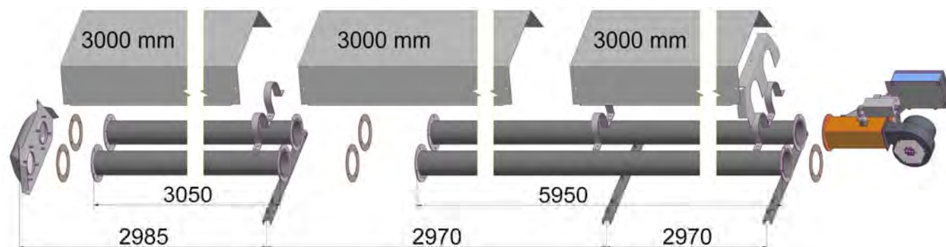
Рисунок 6.3.2.1 Монтажная схема ГИИ-ТМ U
