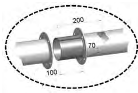
Рисунок 6.3.1 Установка гильзы
