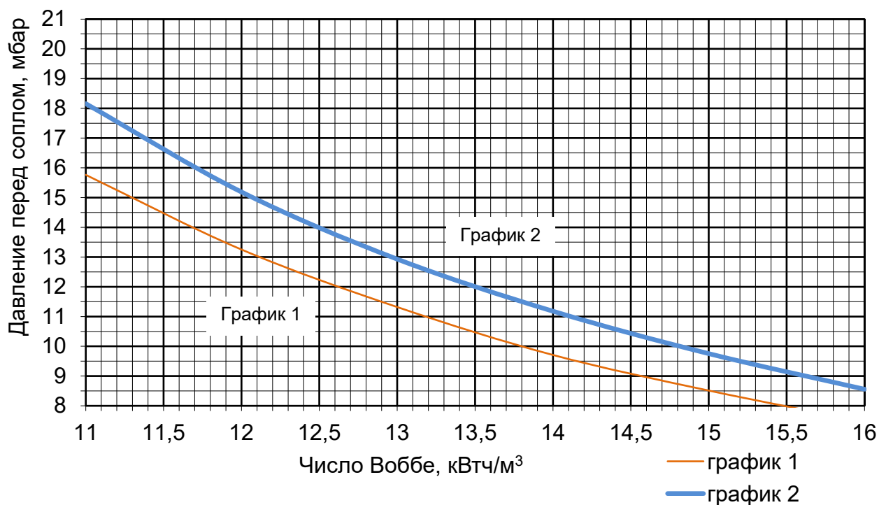
Рисунок 4.3.3 Диаграмма определения давления газа перед соплом
