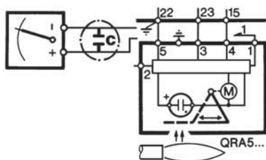
Топочный автомат LGK 16... УФ контроль с QRA 5...
